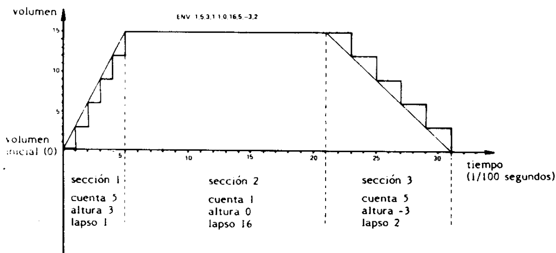
Figura 3: Ejemplo de envolvente de volumen.
