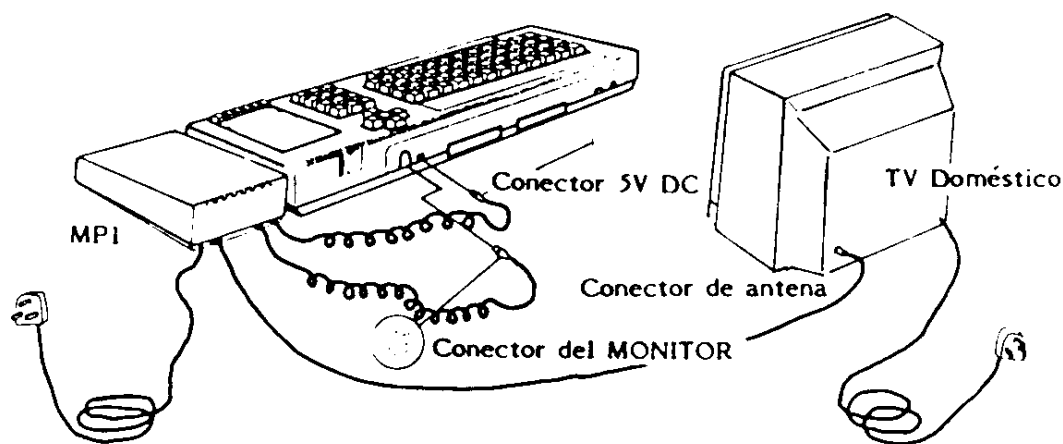
Figura 2: Conexiones para el MPI, ordenador y entrada de antenna en tu TV.
