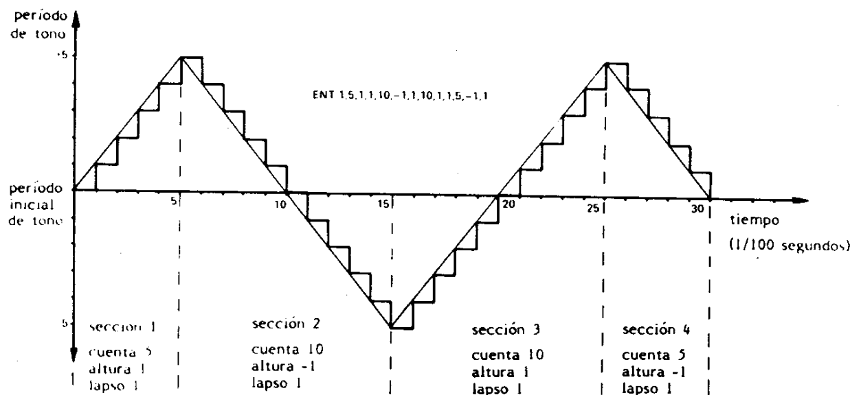
Figura 4: Ejemplo de envolvente de tono.
