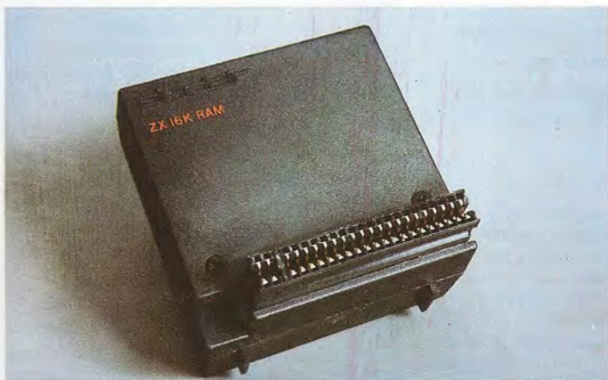
La zona de memoria RAM (1K en la versión estándar) puede ampliarse a partir de la conexión al bus del sistema de módulos adicionales. En la fotografía aparece un módulo compacto de 16 Kbytes de memoria RAM.
