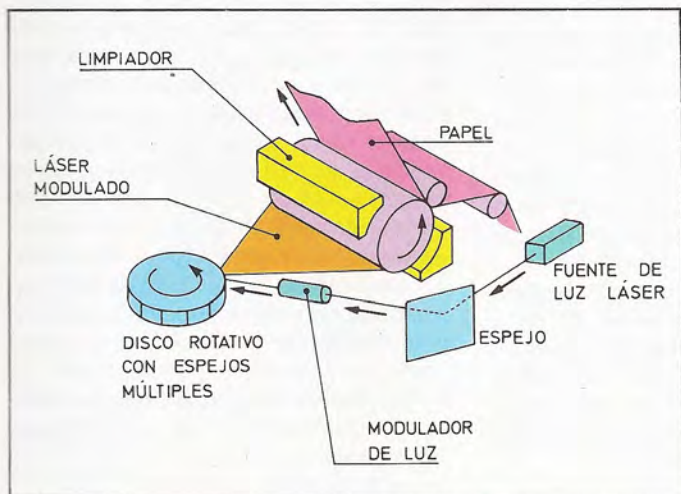
Las impresoras a láser poseen un mecanismo de estampación de relativa complejidad, mecanismo que es gobernado por un rayo láser de baja potencia.
