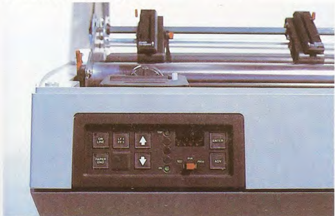
Los modelos de impresora MT 440 disponen de las opciones de arrastre de papel por doble tractor, fricción, inserción frontal e introductor de hojas.
