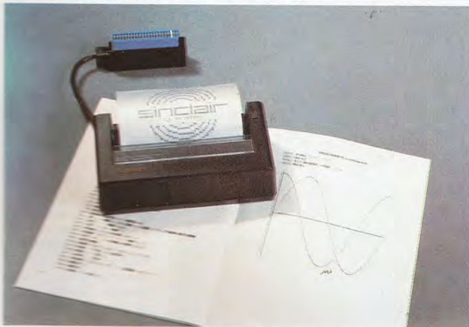
El Spectrum admite la impresora diseñada por Sinclair para su antecesor el ZX-81. Esta microlimpresora de 50 cps imprime sobre papel metalizado hasta un máximo de 32 caracteres por línea.
