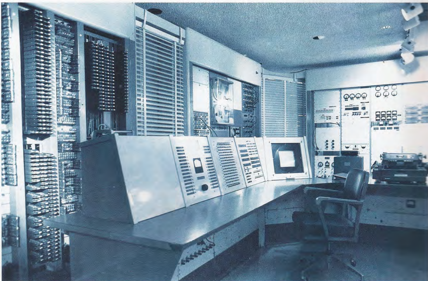
El MIT Lincoln Laboratory TX-0 fue el primer ordenador transistorizado con programa residente. Sus innovaciones más importantes se centraban en el tubo de rayos catódicos, el lápiz óptico y la memoria.
