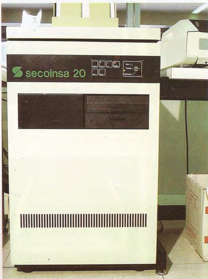
La unidad central se aloja en un mueble vertical, junto con dos unidades de disco (flexible de 8 pulgadas o rígido), la fuente de alimentación y las tarjetas para la expansión del sistema.
