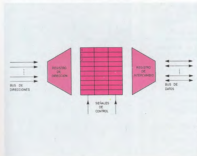
Estructura típica de una unidad de memoria RAM. Obsérvese que en este tipo de memorias (de lectura y escritura) los datos pueden entrar o salir de la unidad a través del correspondiente bus de datos.
