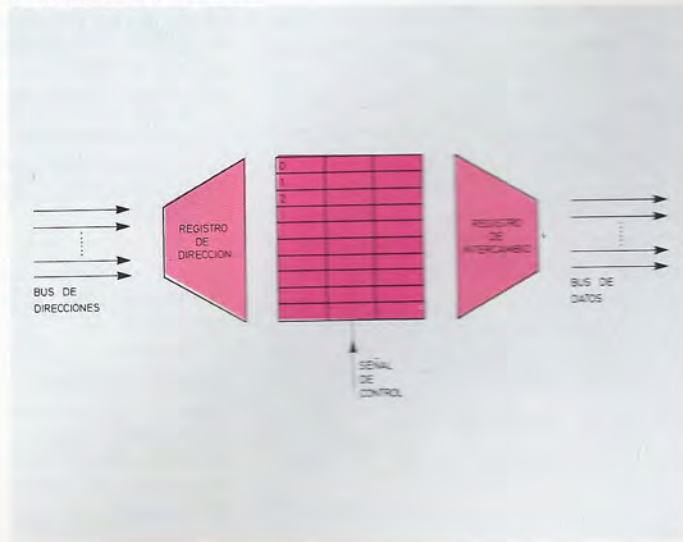
Organización de una unidad de memoria ROM. Dada su característica de memoria de solo lectura, los datos se canalizan sólo en un sentido: del interior de la memoria hacia el exterior a través del bus de datos.
