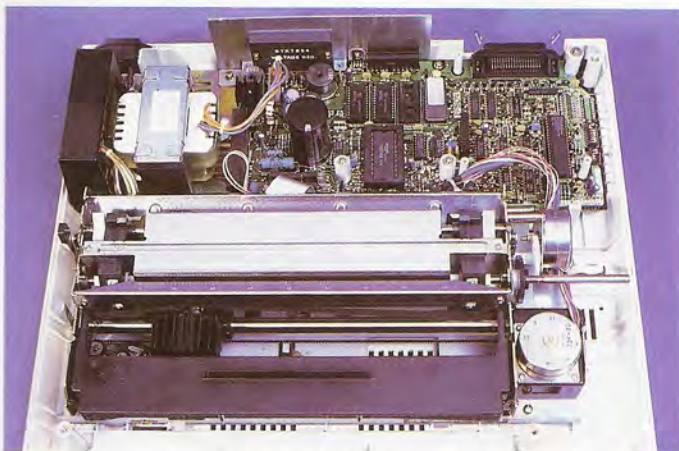
La avanzada tecnología empleada en el diseño de la FX-80, hace que esta impresora posea características tan notables como la posibilidad de impresión de gráficos con sistemas de densidades de puntos; densidades que van desde los 480x8 ó 480x9 puntos por línea, hasta los 1920x8 puntos.
