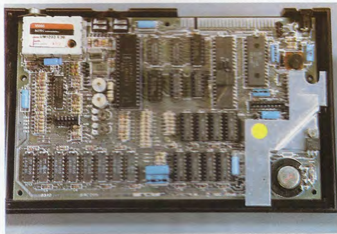
Toda la circuitería electrónica del ZX-Spectrum está incluida en una sola tarjeta de circuito impreso. El bloque metálico que aparece en la zona superior derecha es el modulador UHF-VHF que permite la conexión directa del equipo a la entrada de antena de un receptor TV-color.
