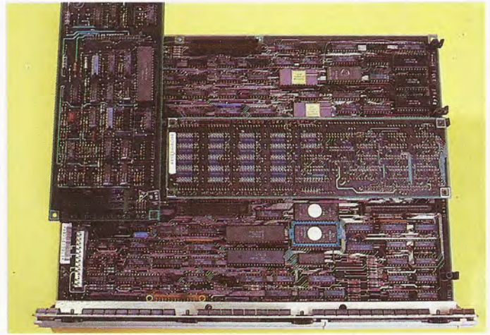
Sobre la tarjeta base está previsto el espacio para alojar las ampliaciones circuitales que admite el sistema: RAM opcional de 64, 128 ó 192 Kbytes, ampliación de comunicaciones, opción para generación de gráficos a color...
