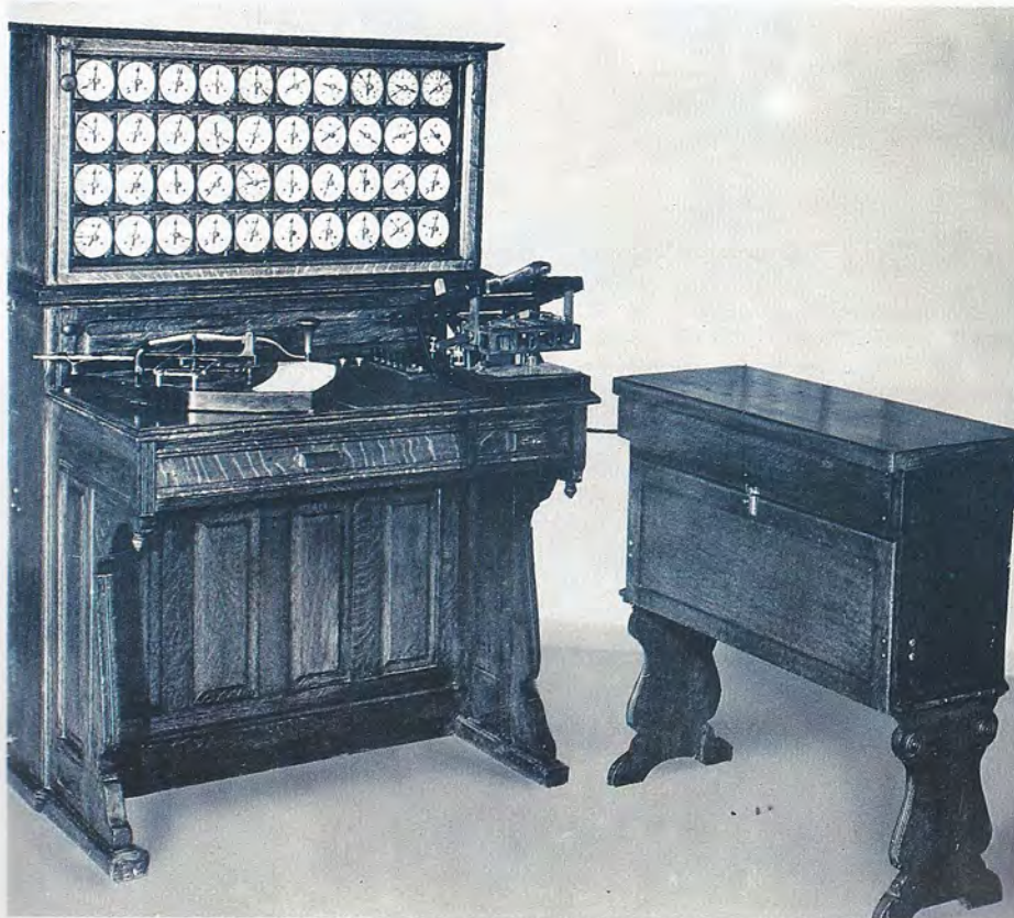
Maquina tabuladora electrica de Hollerith patentada en 1889. Dos veces más veloz que las restantes máquinas contemporáneas, la tabuladora eléctrica es la madre de las modernas máquinas de tratamiento de datos. Se utilizó en 1890 para elaborar el censo de los Estados Unidos de América.
