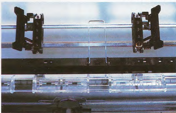
Para el arrastre del papel, las tres versiones de la impresora MT 120 disponen de las siguientes opciones: tractor, fricción o introducción manual.
