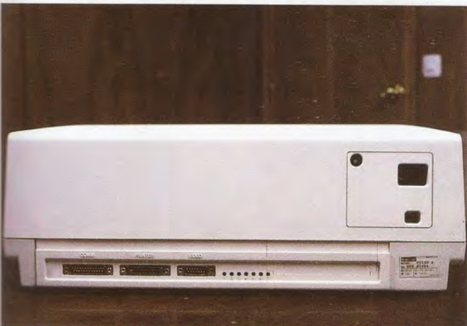
La comunicación periférica del RAINBOW 100 se establece a través de una salida de tipo serie RS/232C para impresora y un acceso de entrada/salida para comunicaciones sincronas o asincronas a nivel de byte.
