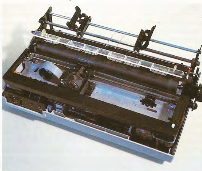
La velocidad de impresión de la MT 120 es de 160 c.p.s., imprimiendo de forma bidireccional optimizada a 80 columnas de ancho.
