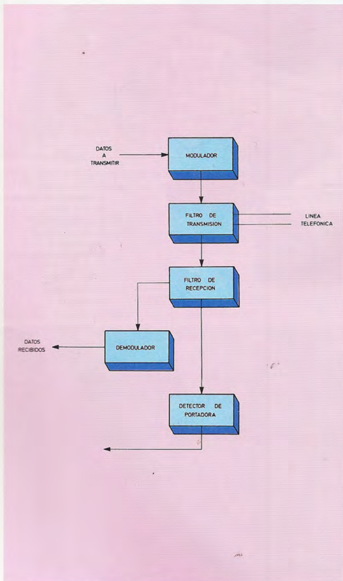
Diagrama de bloques de un modem. Las zonas moduladora y demoduladora realizan las funciones de emisión y recepción de datos, respectivamente.
