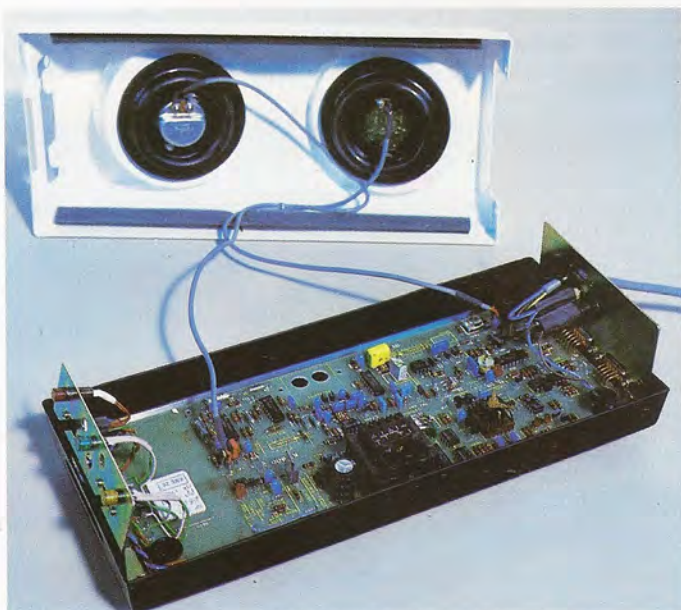
El tipo más común de modems emplea la técnica de modulación FSK. La velocidad de transmisión se selecciona normalmente por medio de microinterruptores internos.
