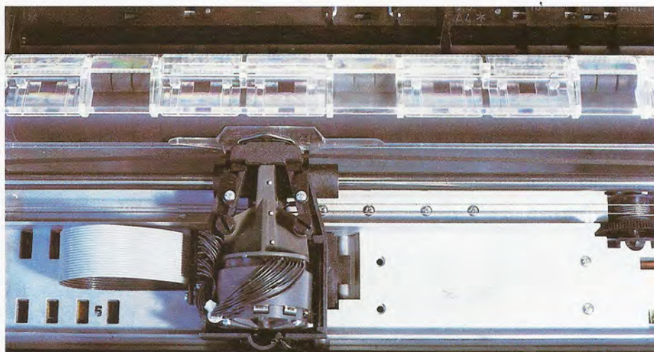
Las tres versiones de la MT 120 difieren en las características de la matriz de agujas. En la versión MT 120 I la matriz es de 9 x 7, en la versión D de 9 x 9 agujas y en la versión L la matriz es seleccionable a 9 x 7 ó 18 x 40.
