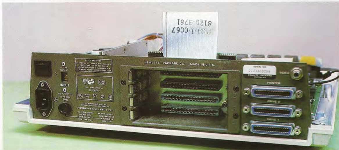
El sistema se presenta en dos versiones: HP-86A y HP-86B, siendo este último modelo de mayor capacidad de memoria y con mayor potencia operativa.
