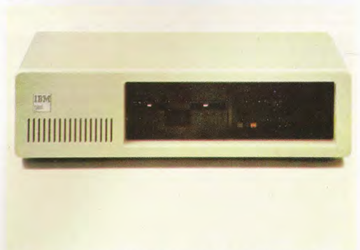
La unidad central del IBM-PC está basada en el microprocesador 8088 e incorpora, en la versión básica, 64 Kbytes de memoria RAM y 40 Kbytes de ROM. El mueble dispone de espacio reservado para la inclusión de dos unidades de disco flexible o una unidad de disco flexible y un disco rígido.
