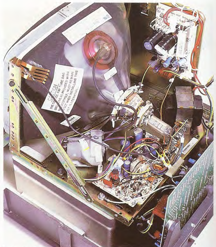
Tanto el teclado como la pantalla y la circuitería electrónica asociada se alojan en una misma caja metálica, cuyas dimensiones son de 43 x 58 x 37 cm.
